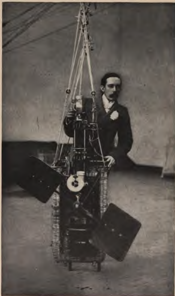
Motor of "No. 1"
